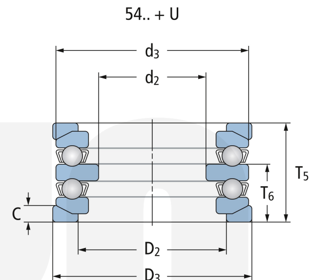
Kugelige Gehäusescheibe + Unterlagscheibe With aligning seat races
