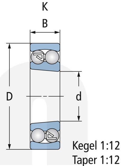
Kegelige Bohrung Tapered bore
