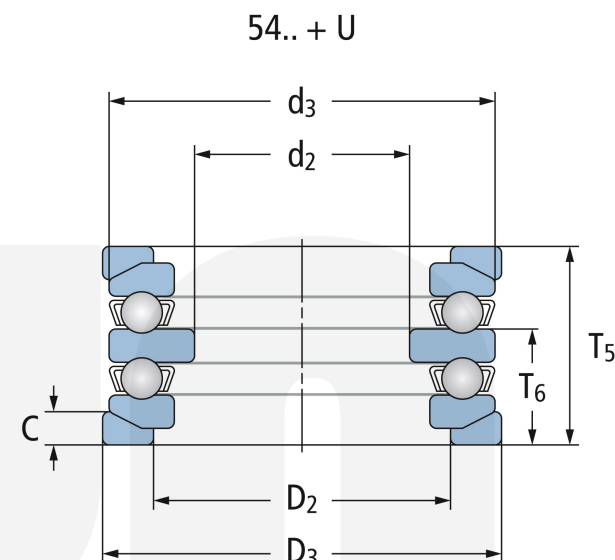
Kugelige Gehäusescheibe + Unterlagscheibe With aligning seat races
