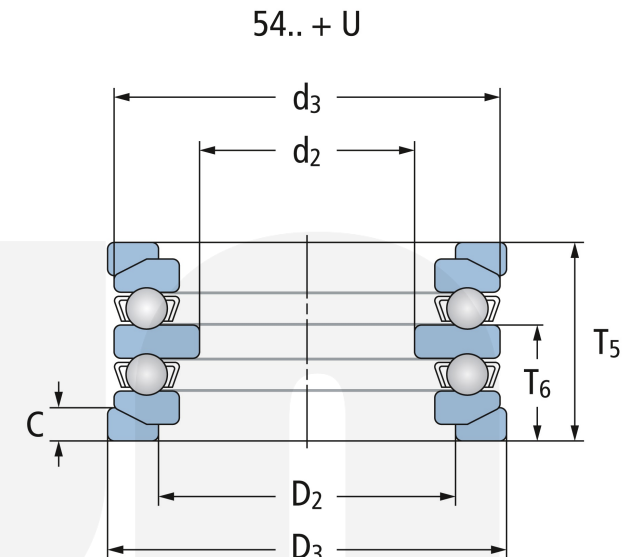
Kugelige Gehäusescheibe + Unterlagscheibe With aligning seat races
