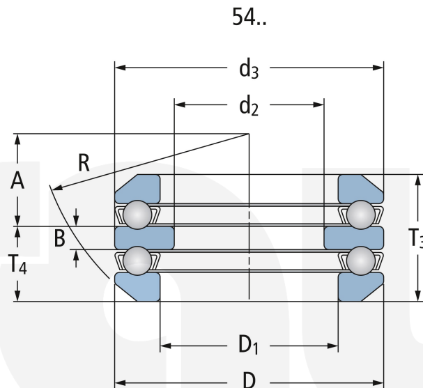
Kugelige Gehäusescheibe With spherical back face
