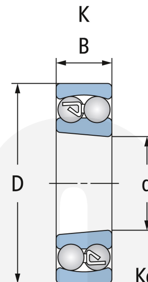
Kegelige Bohrung Tapered bore
