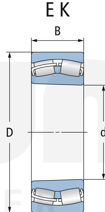
Kegelige Bohrung Tapered bore
