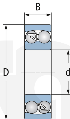
Zylindrische Bohrung offen Cylindrical bore Open
