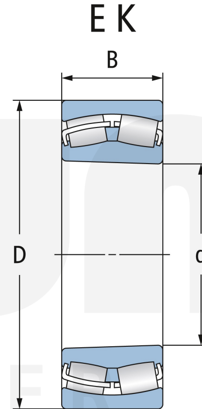
Kegelige Bohrung
