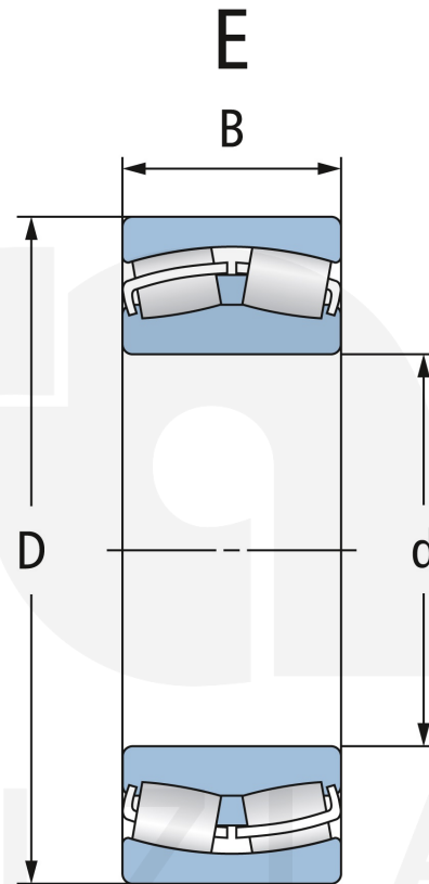
Zylindrische Bohrung
