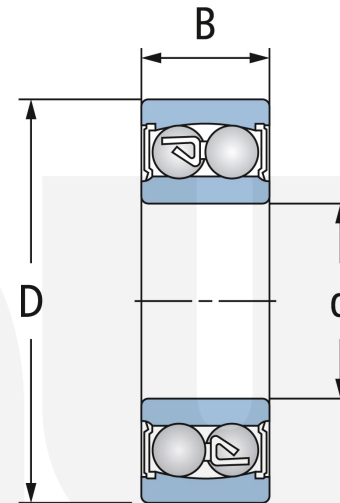
Zylindrische Bohrung abgedichtet - 2RS Cylindrical bore 2RS
