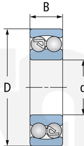
Zylindrische Bohrung offen Cylindrical bore Open
