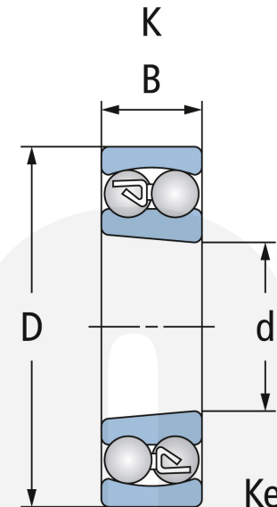
Kegelige Bohrung Tapered bore
